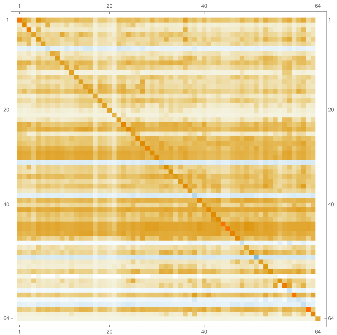
Σχήμα Π1.7. Διάγραμμα της ανά Τομέα Μήτρας Συνολικής Συμβολής των Κερδών
