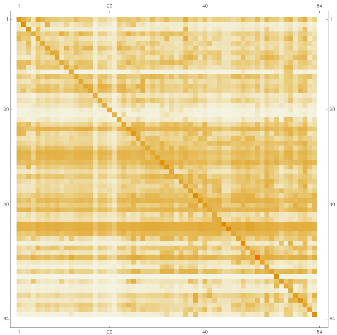
Σχήμα Π1.6. Διάγραμμα της ανά Τομέα Μήτρας Συνολικής Συμβολής των Αποσθέσεων
