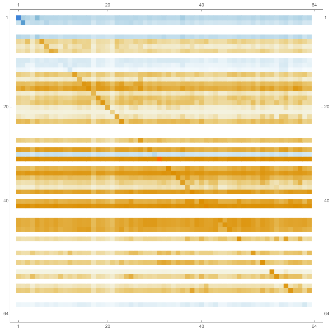
Σχήμα Π1.5. Διάγραμμα της ανά Τομέα Μήτρας Συνολικής Συμβολής των Άλλων Καθαρών Φόρων στην Παραγωγή
