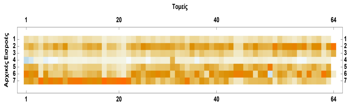
Σχήμα 1. Διάγραμμα της μήτρας C
