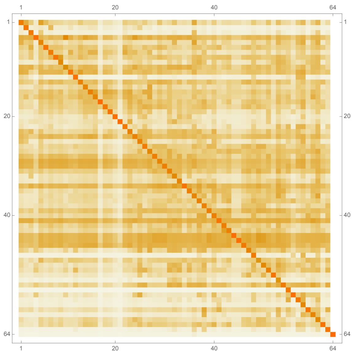
Σχήμα Π1.1. Διάγραμμα της ανά Τομέα Μήτρας Συνολικής Συμβολής των Αρχικών Εισροών
