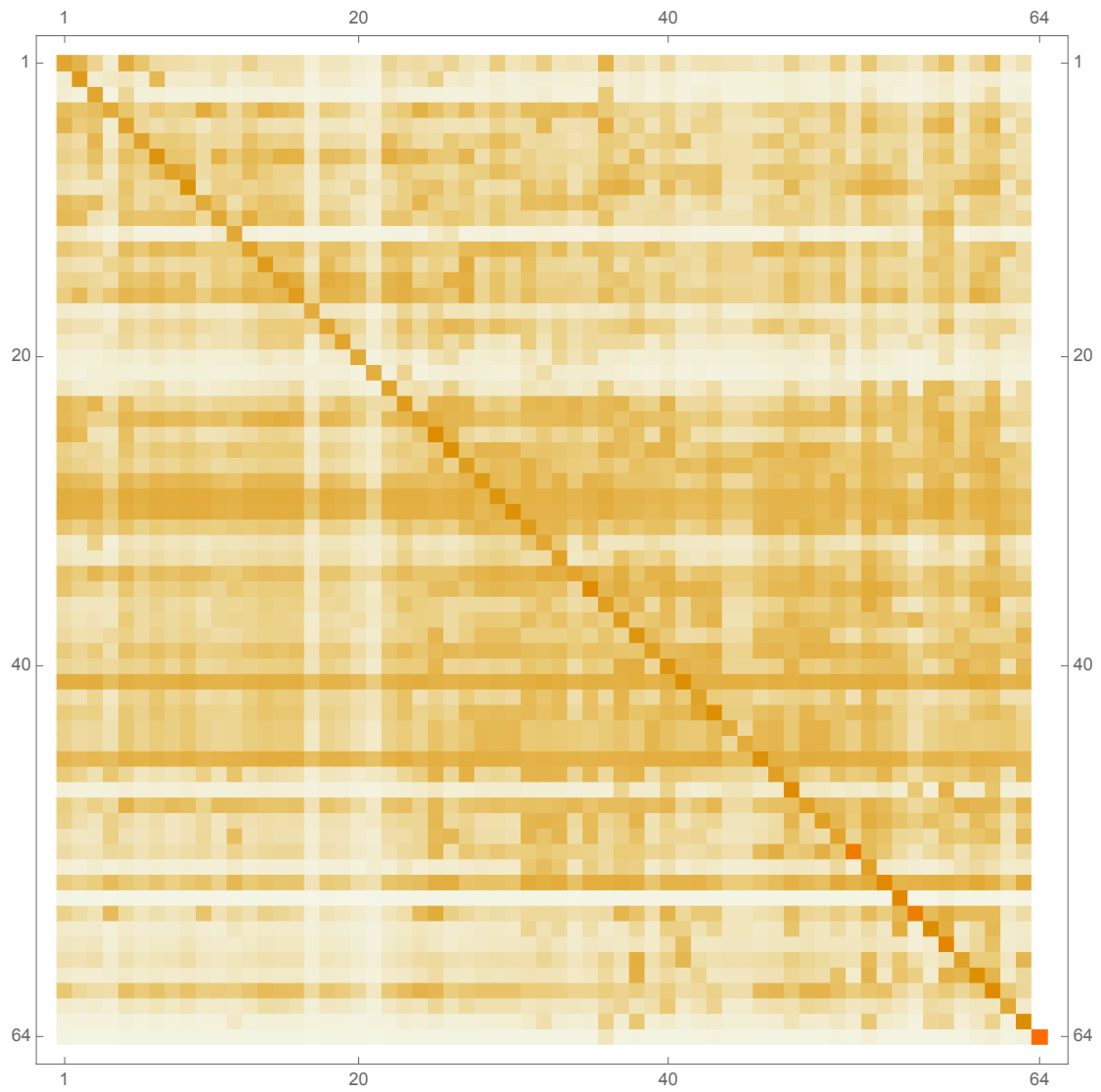
Σχήμα Π1.3. Διάγραμμα της ανά Τομέα Μήτρας Συνολικής Συμβολής των Μισθών
