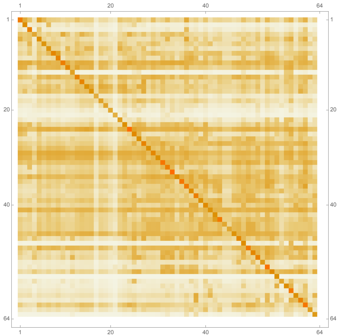
Σχήμα Π1.2. Διάγραμμα της ανά Τομέα Μήτρας Συνολικής Συμβολής των Καθαρών Φόρων Προϊόντων
