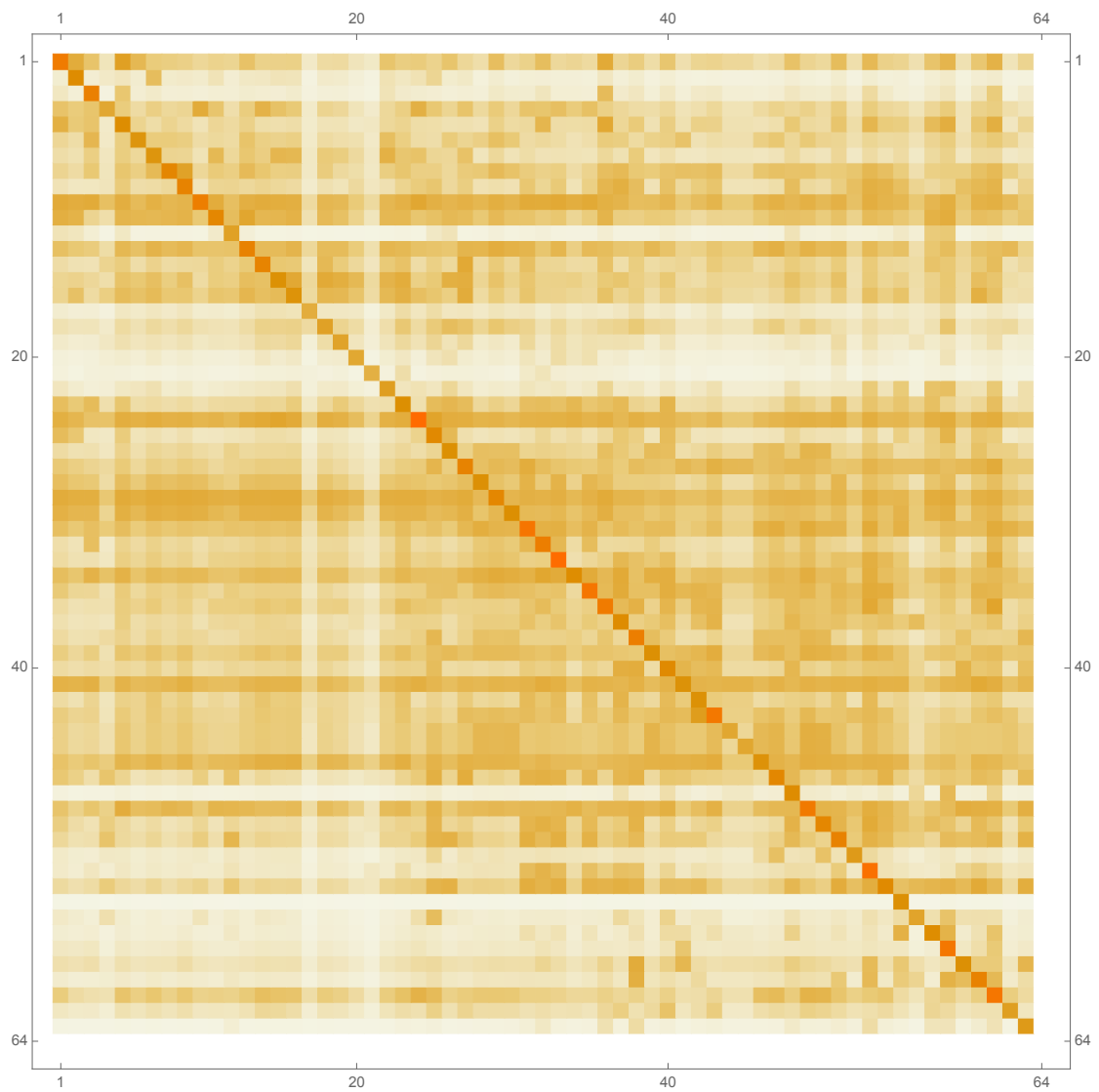
Σχήμα Π1.4. Διάγραμμα της ανά Τομέα Μήτρας Συνολικής Συμβολής των Εργοδοτικών Εισφορών
