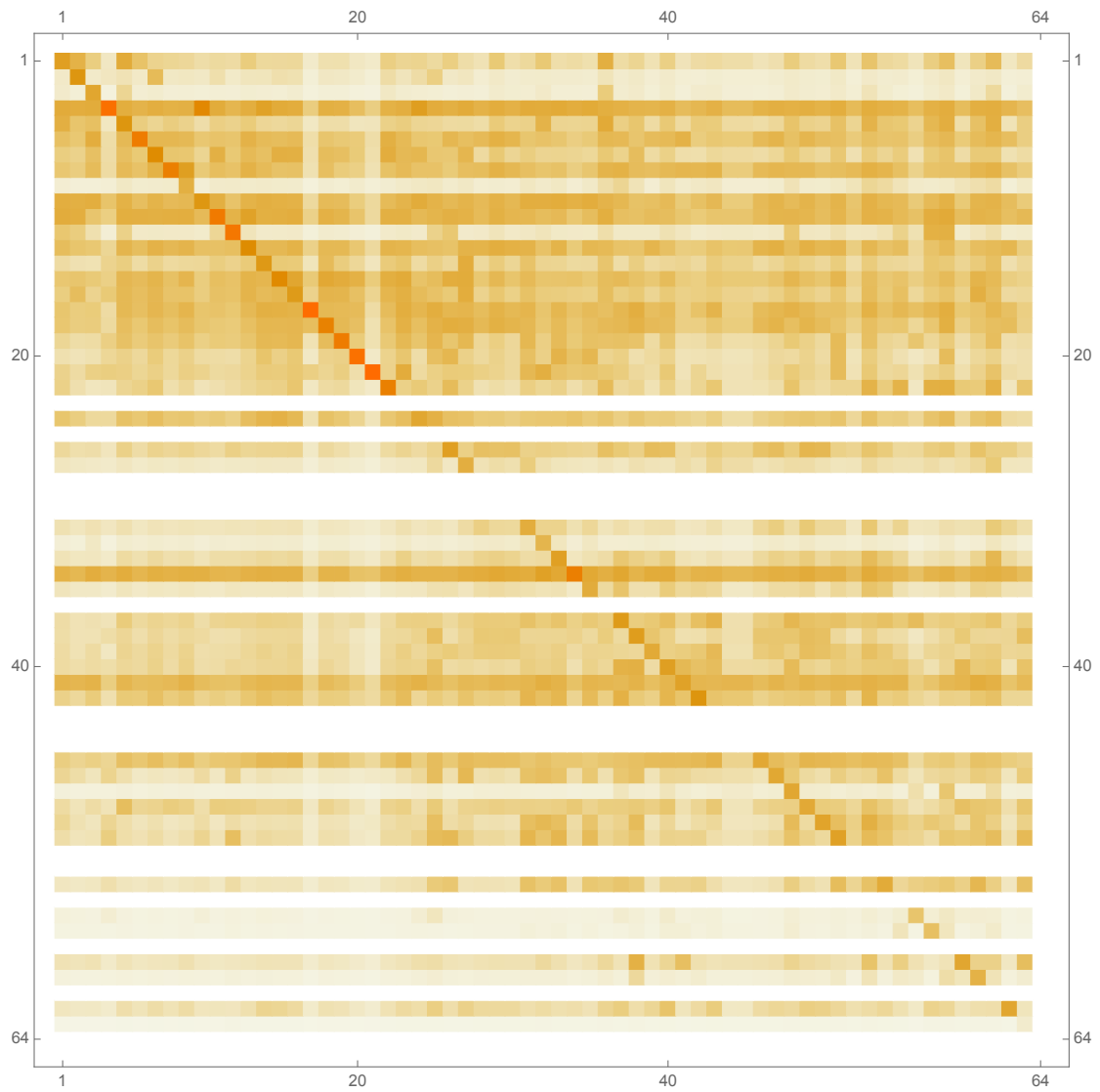
Σχήμα Π1.8. Διάγραμμα της ανά Τομέα Μήτρας Συνολικής Συμβολής των Εισαγωγών
